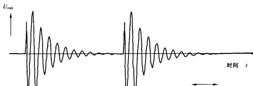
图 E1. b 带宽 \Delta f = 45\ \text{kHz} \sim 440\ \text{kHz} , 长时输入脉冲
