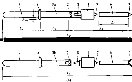
图 1 验电器
