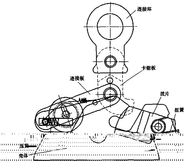
图2 绳索式防坠器典型结构和主要零部件示意图
