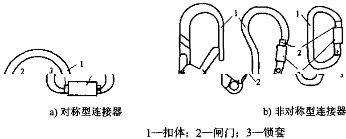
图3 连接器结构示意图
