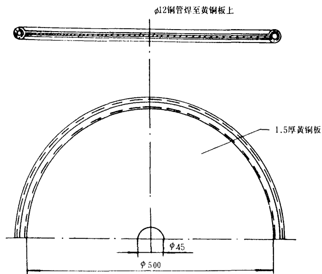
图 A2 电极结构示意图(两个侧面)
